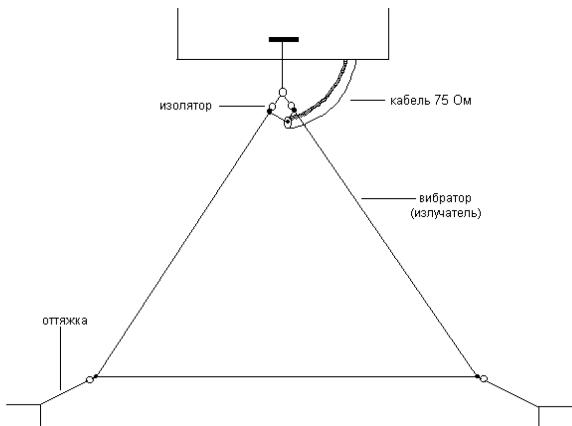
Рис.2.13. Антенна «треугольник»
