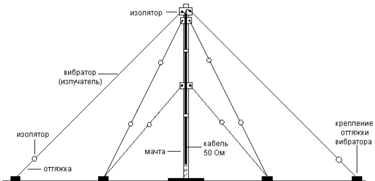
Рис.2.12. Антенна «Inverted V»
