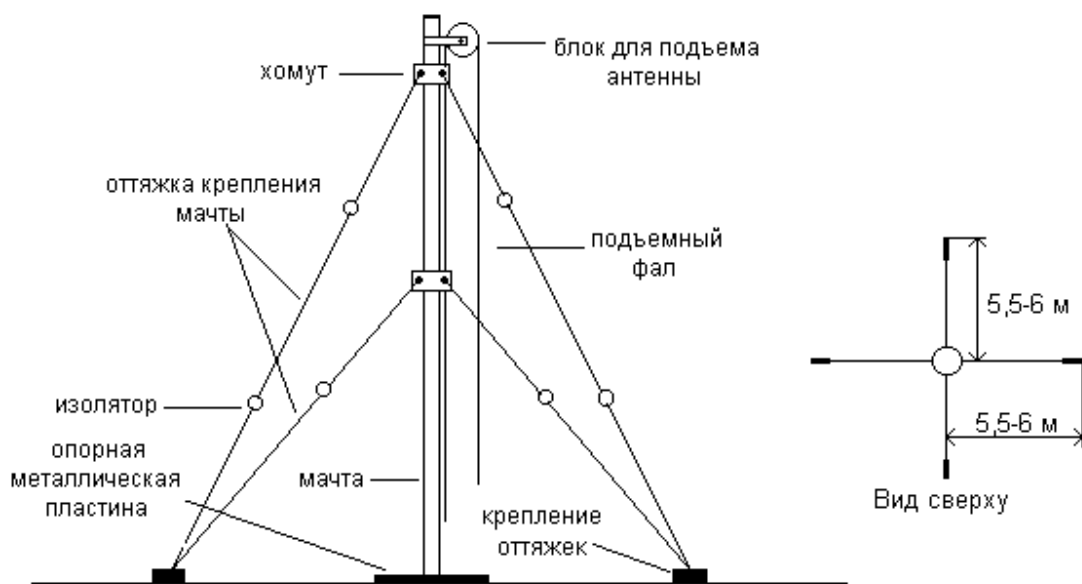
Рис.2.9. Антенная мачта в развернутом виде
