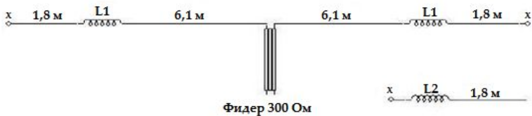
Рис.2.15. Антенна «укороченный диполь»
