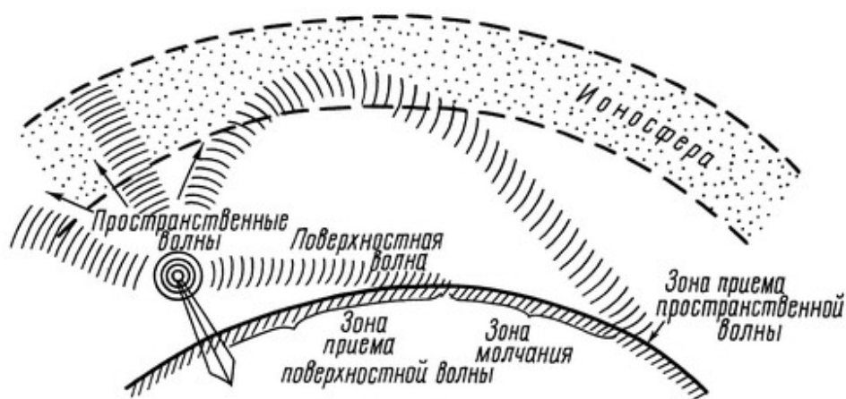
Рис.2.1. Распространение радиоволн
