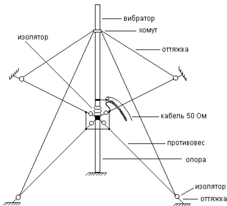
Рис.2.14. Антенна «граунд-плэйн»
