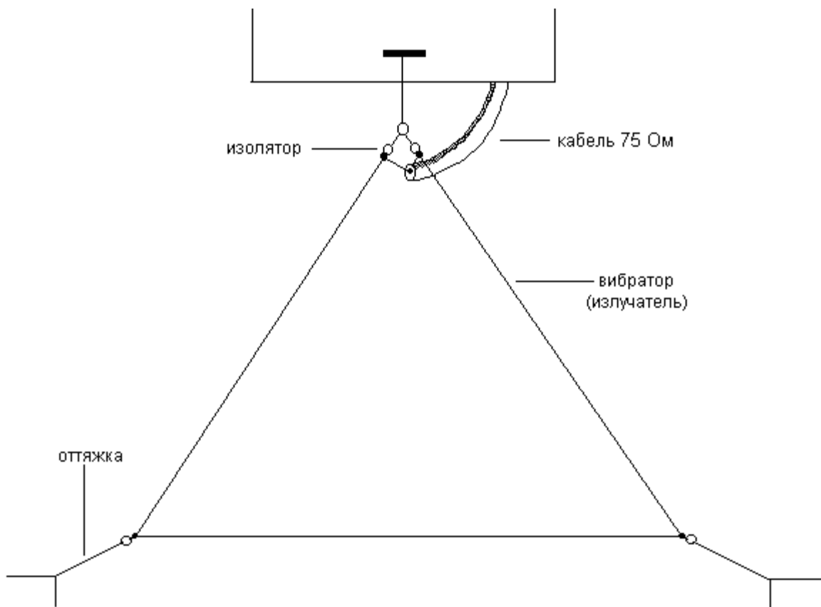
Рис. 2.12. Антенна «треугольник»
