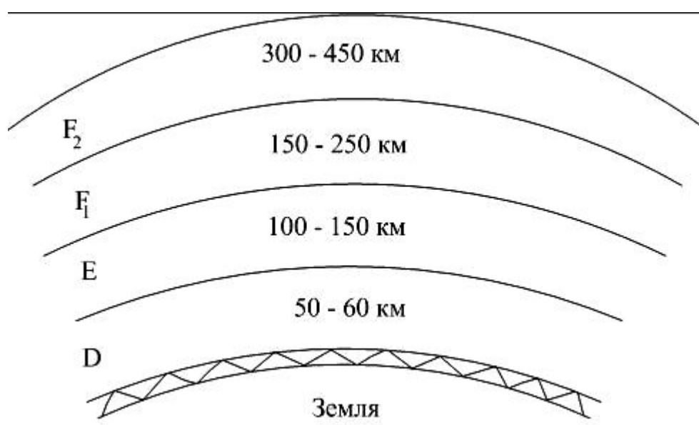
Рис. 2.2. Ионосферные слои
